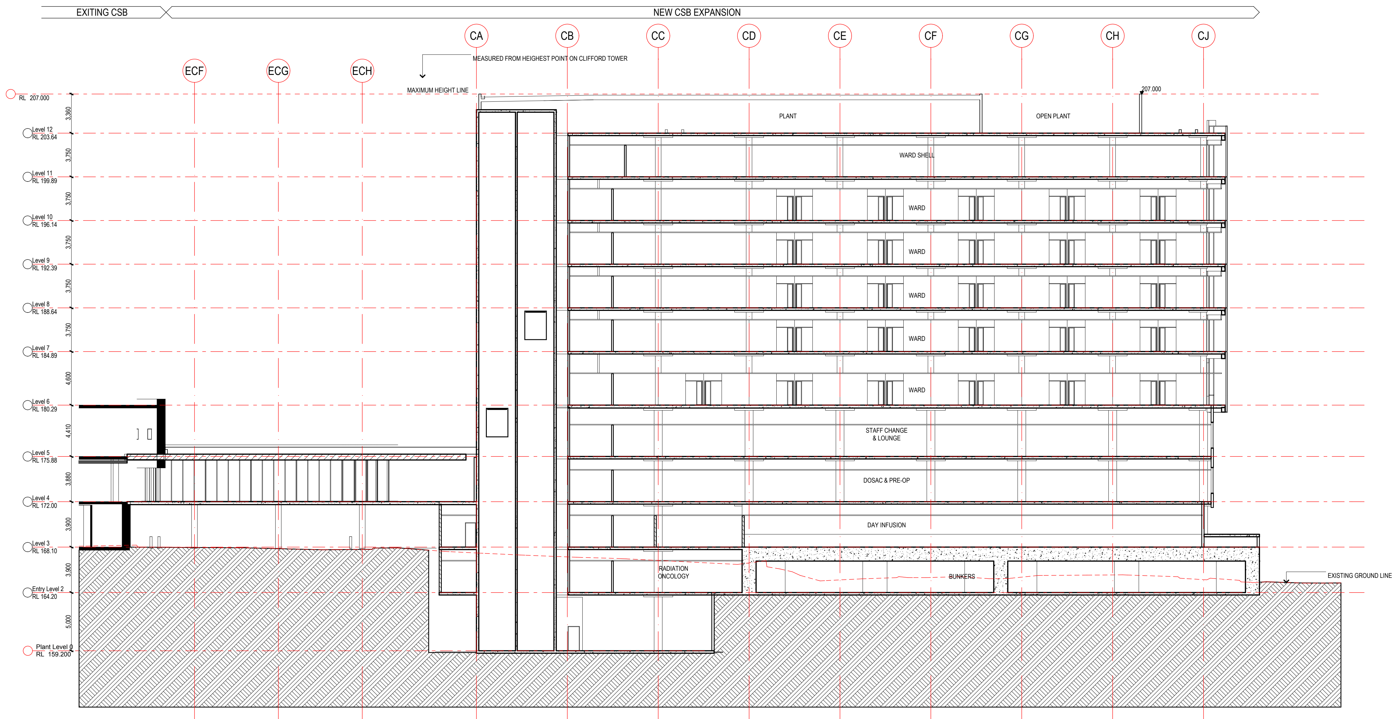
C-E SECTION E SCALE 1:200
